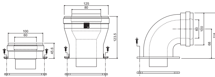
рис. 7 - Элементы для коаксиальных воздуховодов
