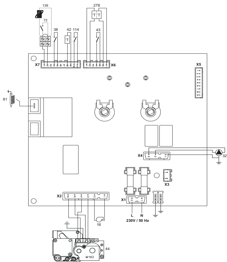
рис. 16 - Электрическая схема
