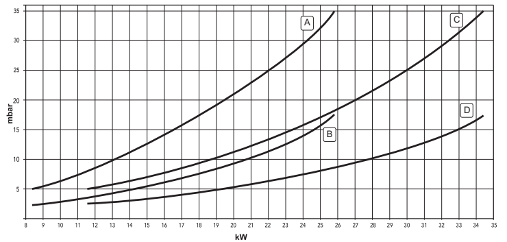
рис. 15 - Диаграммы давление - мощность
